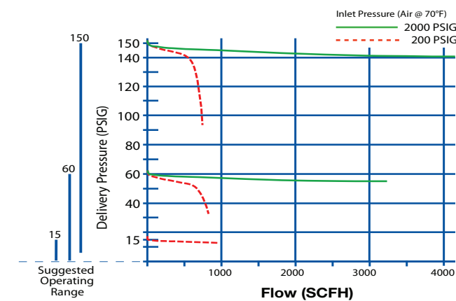
G250 Flow Data
